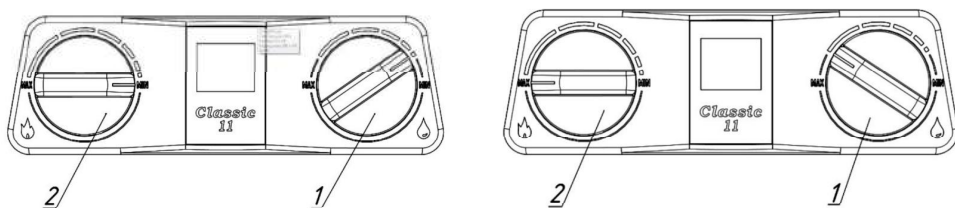
а) Ручки регулировки расхода воды 1 и расхода газа 2 в положении “Минимальный расход” б) Ручки регулировки расхода воды 1 и расхода газа 2 в положении “Максимальный расход”
