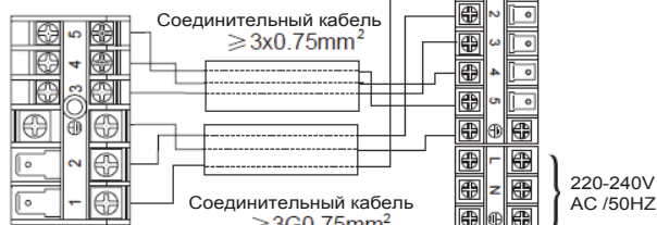
Внутренний блок
