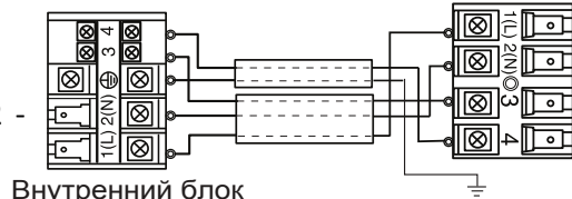
Внутренний блок
